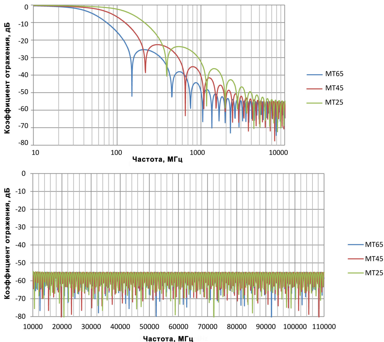
Типичные характеристики поглотителя MT серии (нормальное падение волны)
